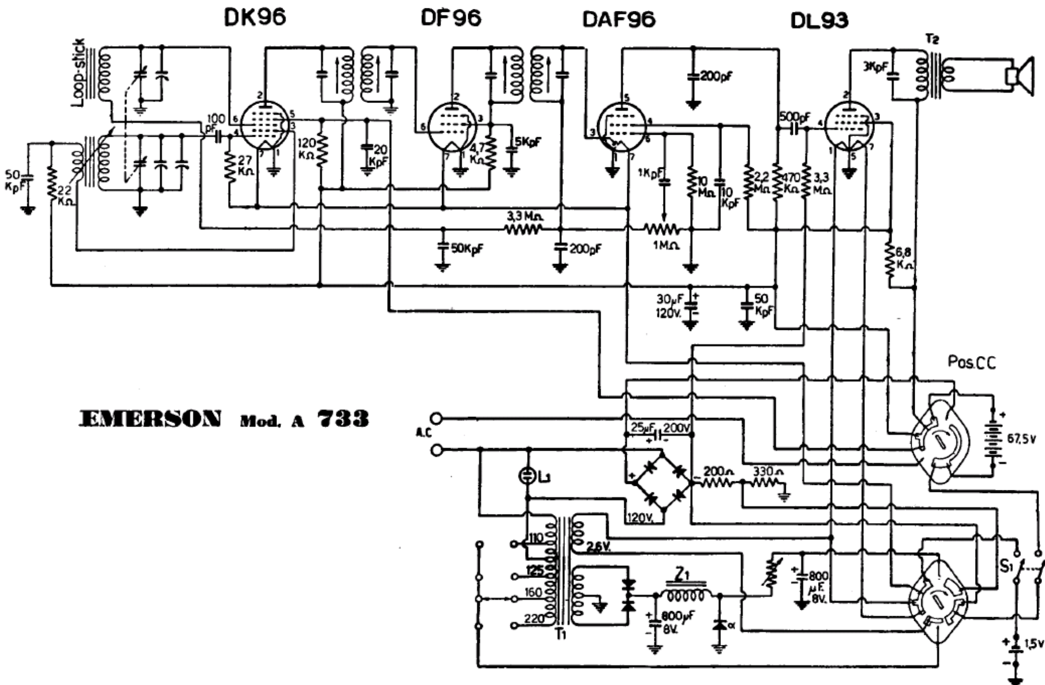
EMERSON-SICART - Mod. Emerson A 733. Apparecchio portatile del tipo pile-rete, a due vie. L'alimentatore anodico e di accensione è incorporato. Commutatore in posizione alimentazione pile. Gamma onde medie con antenna in ferrite. Media frequenza 455 kc/s.
